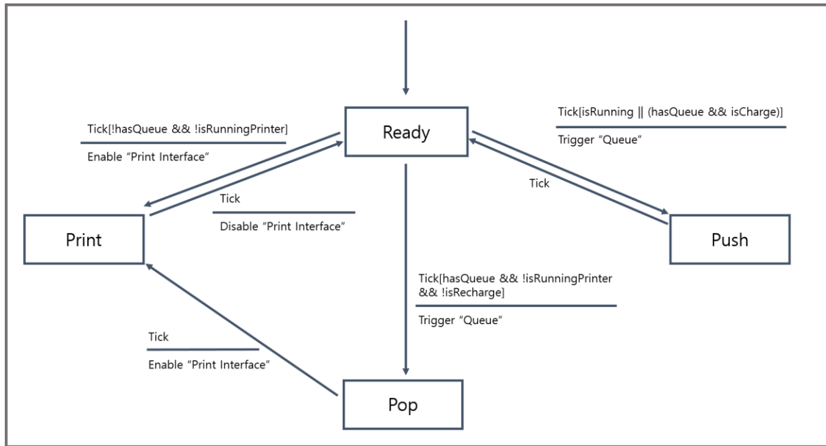
그림 3 NPS Level 4 DFD - Print Manager
