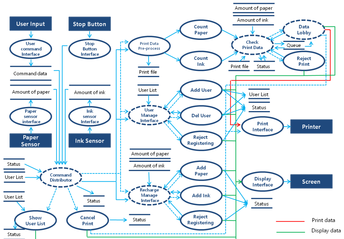
그림 1 NPS Overall DFD
