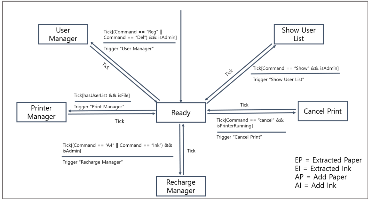
그림 2 NPS Level 3 STD
