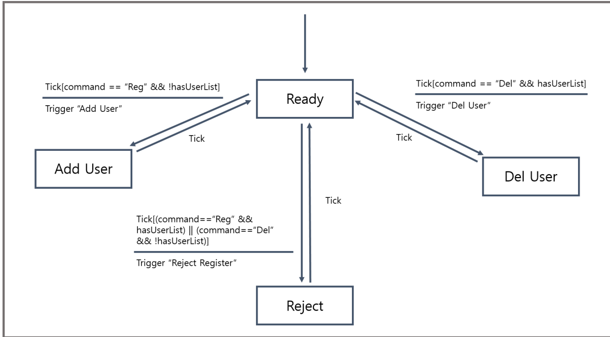
그림 4 NPS Level 4 DFD - User Manager
